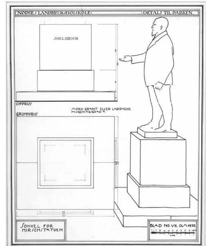
Hirschmonumentet ble plassert i akse fra Tårnbygningen, etter Olav L. Moens parkplan fra 1924. Moen laget detaljtegningen til sokkelen. Han ønsket denne utført i en mørk steinsort og sokkelen ble utført i grovhugget larvikitt. Tegning Olav L. Moen. Arkiv for norsk landskapsarkitektur, NMBU.
